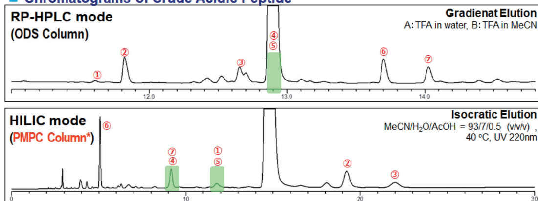
図7 Acidic peptide中の不純物分析(上段：ODSカラム，下段：PMPCカラム)
